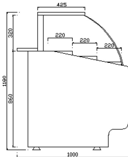
Lada pralinowa LP-95 S-3P
