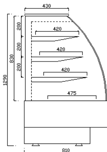
Lada cukiernicza LC-95 S/PM
