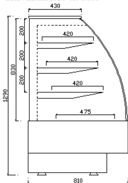
Lada cukiernicza LC-135 S/PM
